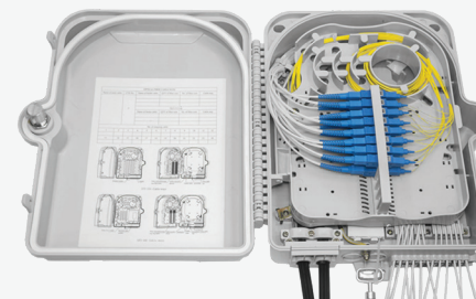
FTTH распределительные коробки
